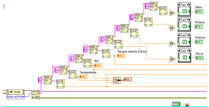
Figura 6 Lectura de puerto serial
